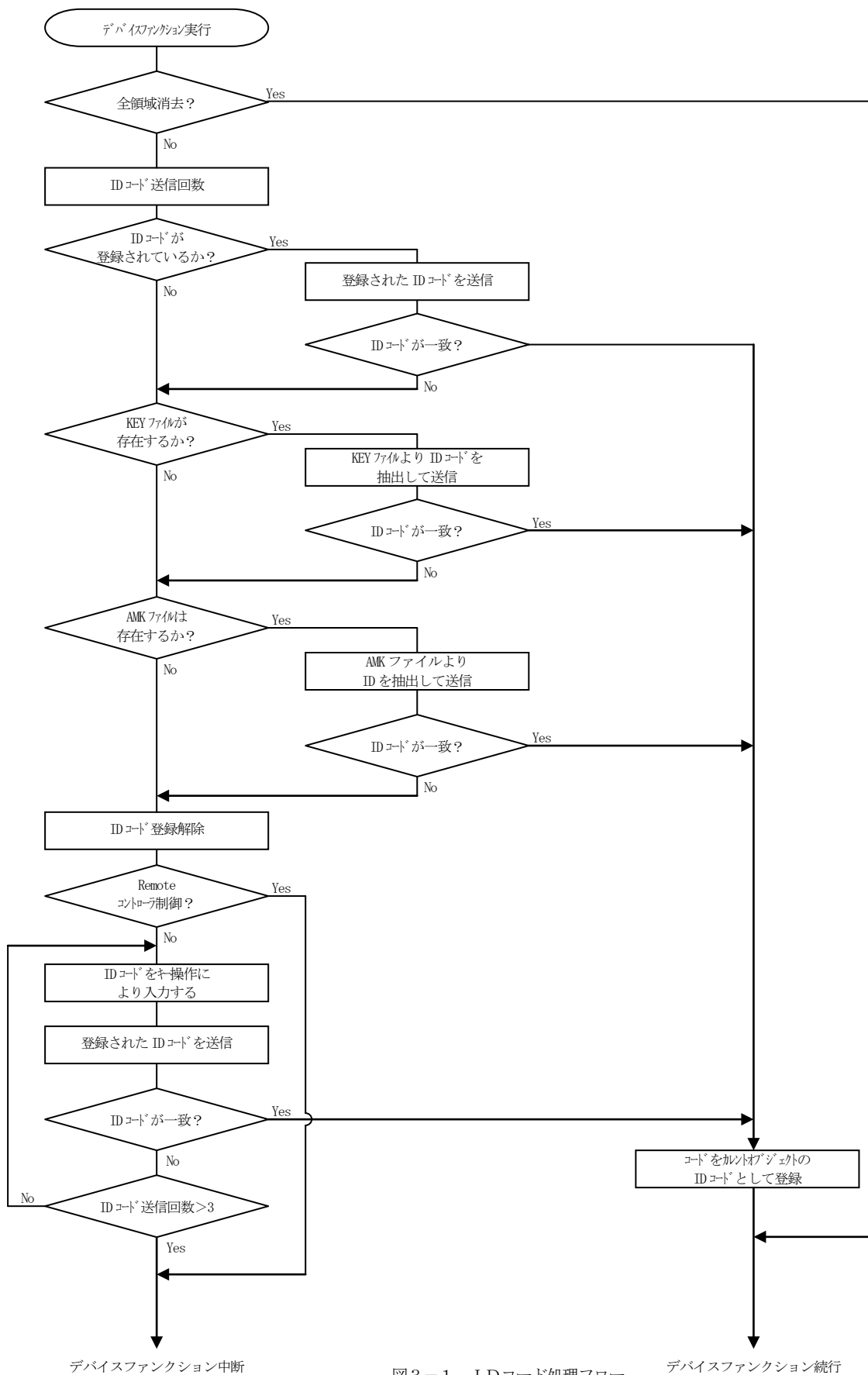
図3-1. IDコード処理フロー
